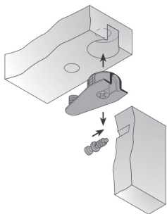
Стяжка эксцентриковая, усиленная
