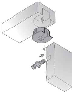
Стяжка эксцентриковая в пластиковом корпусе
