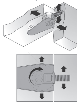
Фиксация стяжки
