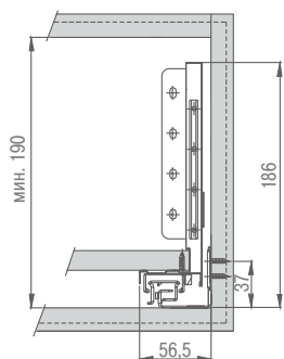
Установочные размеры ящика
