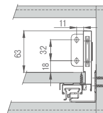
Присадочные размеры для задней стенки
