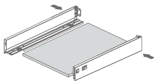
2. Установка дна ящика
