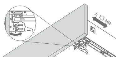
Регулировка угла наклона фасада + 1,5 мм
