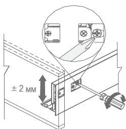
Регулировка фасада по высоте + 2 мм
