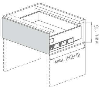
Габариты ящика
