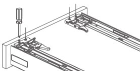
7. Установка креплений к направляющим
