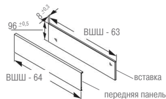
Раскрой вставки для передней панели (изготавливается самостоятельно)
