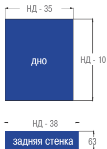
Раскрой ящика
