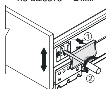
Регулировка по высоте ± 2 мм
