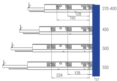
Присадочные размеры направляющих
