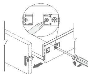
Снятие фасада
