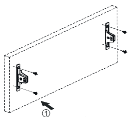
Снятие фасада
