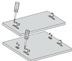
4. Установка креплений к фасаду/ установка креплений релингов
