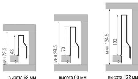
высота 63 мм
