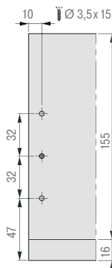
Установочные размеры для задней стенки
