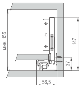
Установочные размеры ящика
