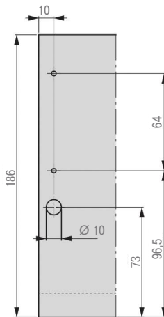
Установочные размеры для задней стенки
