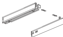
1. Установка креплений задней панели на боковины
