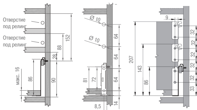
Присадочные размеры для задней стенки
