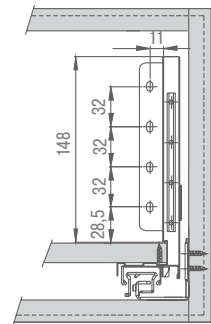
Присадочные размеры для задней стенки
