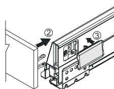
Регулировка по высоте ± 2 мм
