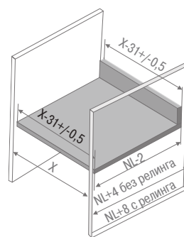
Установочные размеры
