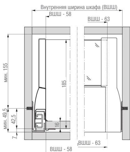
Установочные размеры для фасада
