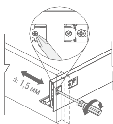
Регулировка фасада вправо + 1,5 мм/ влево + 1,5 мм
