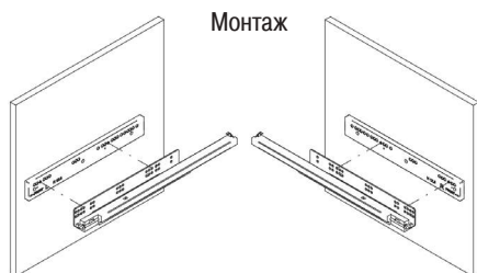
Монтаж
