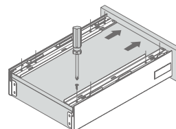
6. Фиксация боковин к дну
