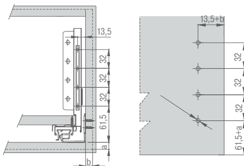
Присадочные размеры фасада
