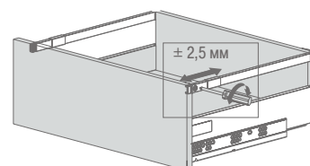
Регулировки для релинга
