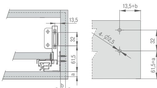
Присадочные размеры фасада
