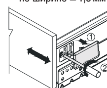
Регулировка по ширине ± 1,5 мм
