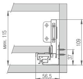
Установочные размеры ящика
