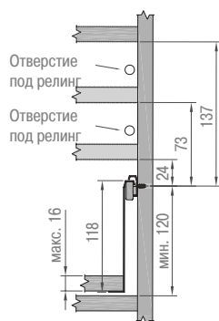
Присадочные размеры для фасада
