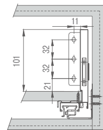
Присадочные размеры для задней стенки
