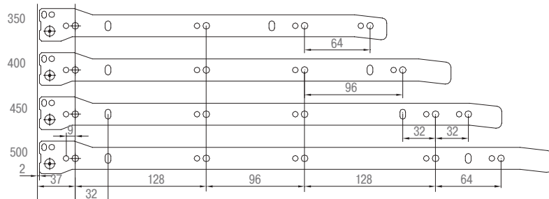
Присадочные размеры для установки направляющих
