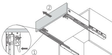
Снятие ящика с направляющих
