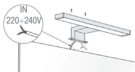
Установка светильника
