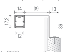
Габаритные размеры
