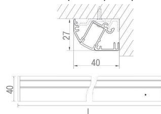
Габаритные размеры
