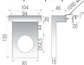
Установка светильника
