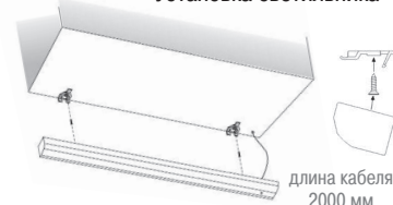
Установка светильника
