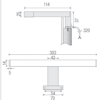
Установка светильника
