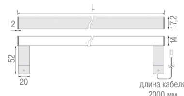
Установка светильника
