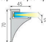
Габаритные размеры
