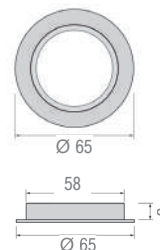
Габаритные размеры
