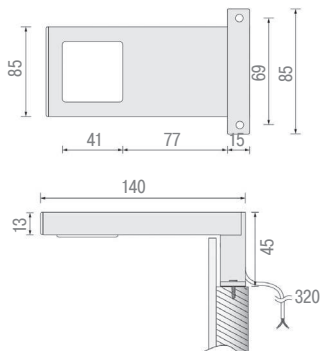
Установка светильника
