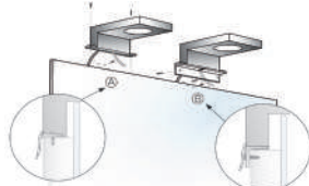
Установка светильника
