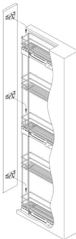
Установка фасада
