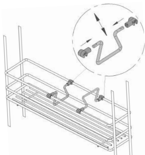
Установка делителей
