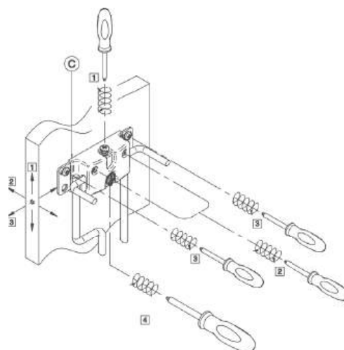
Регулировка фасада
