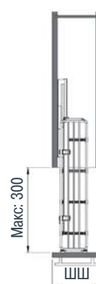
Левое расположение
