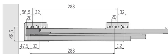
Присадочные размеры для установки направляющих NOVA PRO для решетчатой емкости GALAXY
