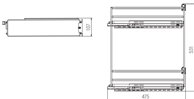
Габаритные размеры
