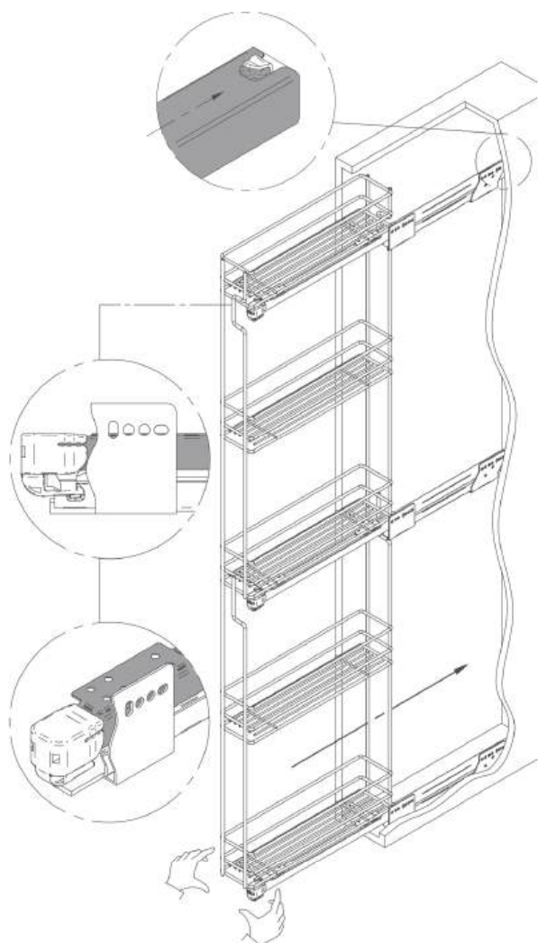
Установка делителей
