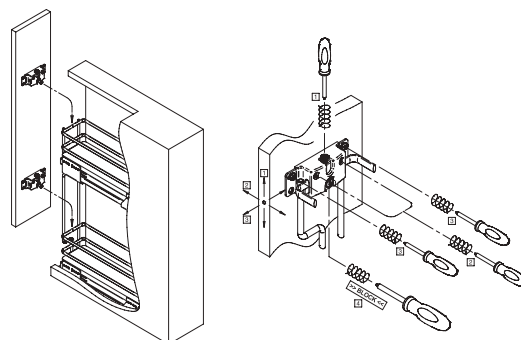
Установка и регулировка фасада
